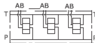
Hydraulické schéma
