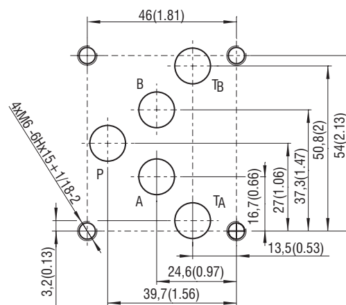
Kanály P, A, B, T - max. \varnothing 11,2 mm (0.44 in)
