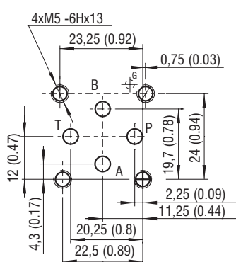
ISO 4401-02-01-0-05
